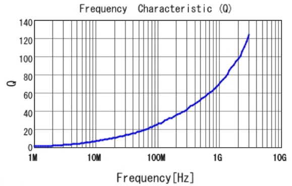
■ LQW15AN2N4B8Z Q
