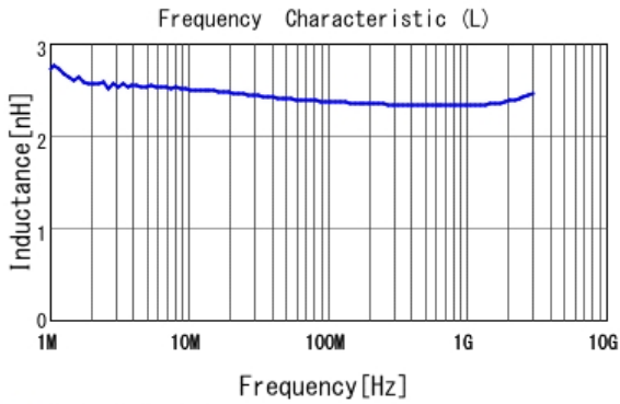
■ LQW15AN2N4B8Z L
