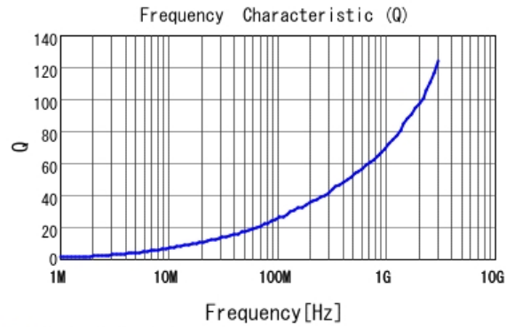
■ LQW15AN2N4B80 Q
