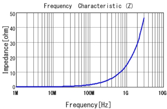
■ LQW15AN2N4B80 |Z|
