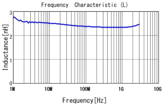
■ LQW15AN2N4B80 L
