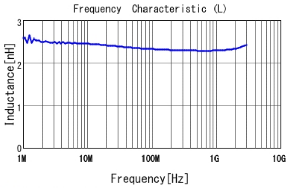
■ LQW15AN2N3G80 L
