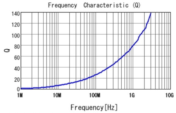
■ LQW15AN2N3G80 Q
