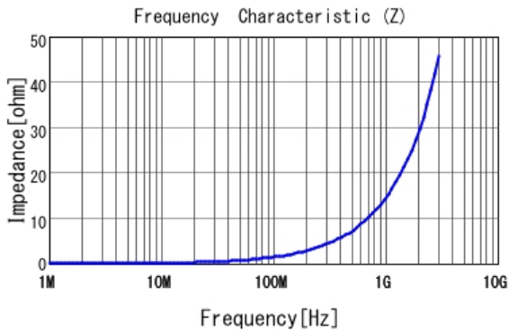
■ LQW15AN2N3G80 |Z|
