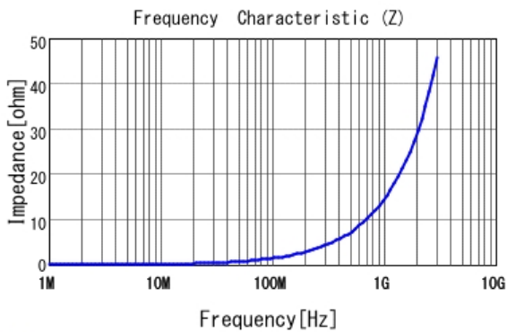
■ LQW15AN2N3B80 |Z|
