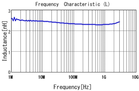
■ LQW15AN2N3B80 L
