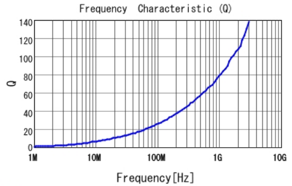
■ LQW15AN2N3B80 Q
