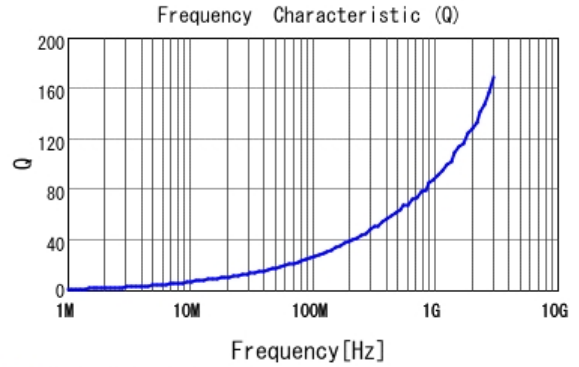
■ LQW15AN2N2G8Z Q
