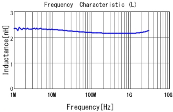
■ LQW15AN2N2G8Z L
