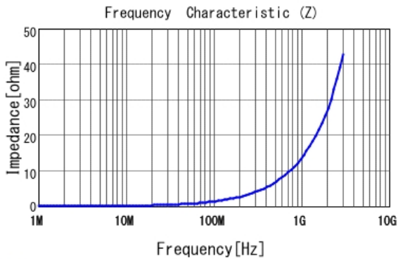
■ LQW15AN2N2G8Z |Z|
