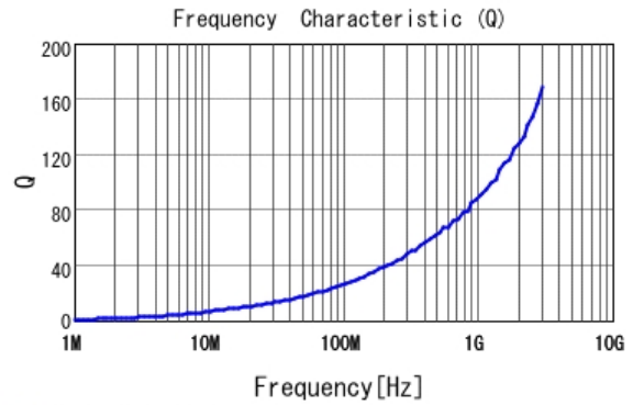
■ LQW15AN2N2C80 Q
