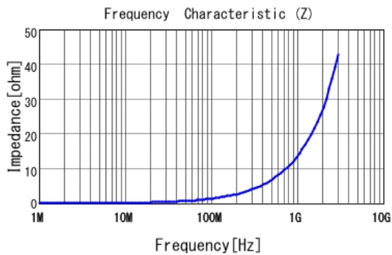
■ LQW15AN2N2C80 |Z|
