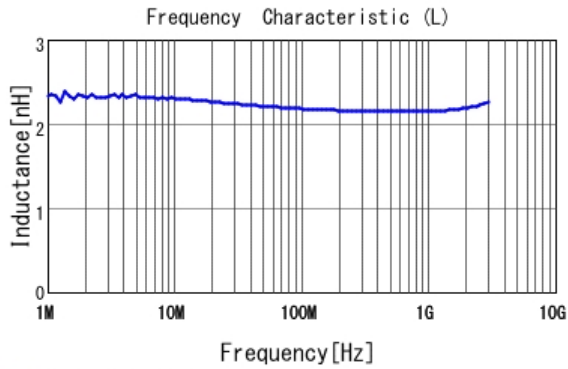
■ LQW15AN2N2C80 L
