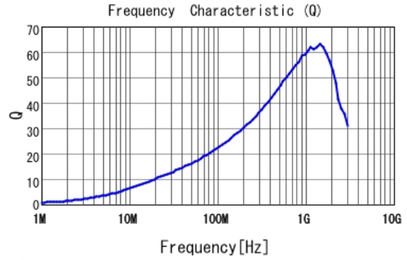
■ LQW15AN27NG8Z Q
