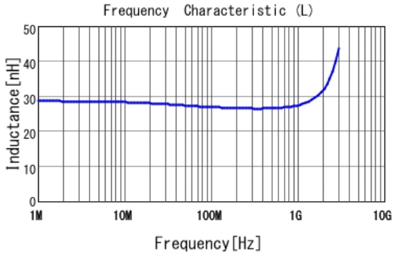
■ LQW15AN27NG8Z L
