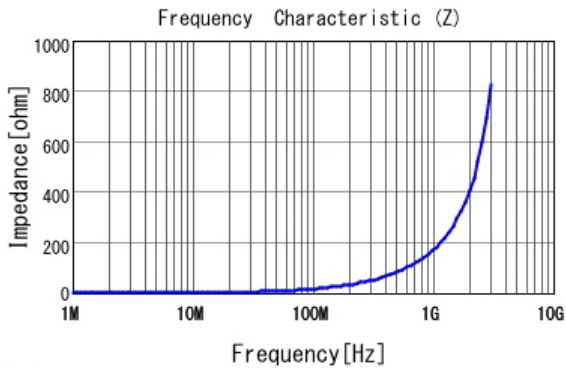
■ LQW15AN27NG80 |Z|
