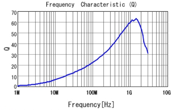
■ LQW15AN27NG80 Q
