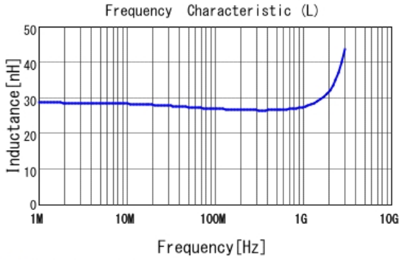
■ LQW15AN27NG80 L
