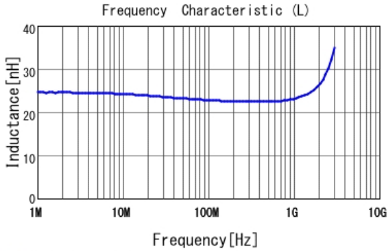
■ LQW15AN23NG80 L
