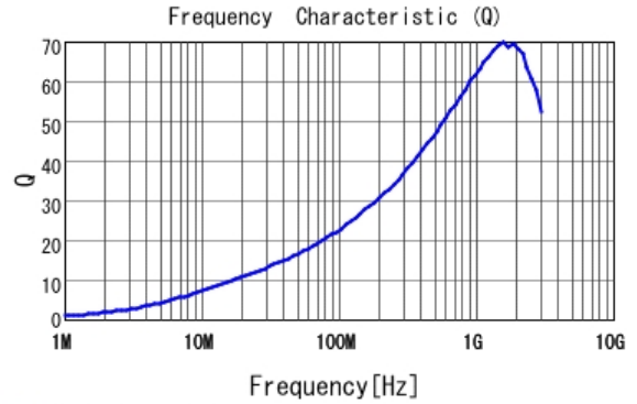
■ LQW15AN23NG80 Q
