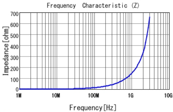
■ LQW15AN23NG80 |Z|
