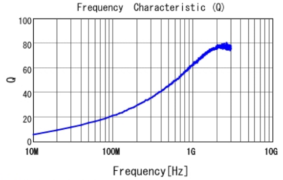
■ LQW15AN22NJ0Z Q
