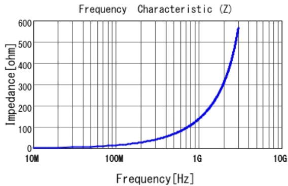
■ LQW15AN22NJ0Z |Z|
