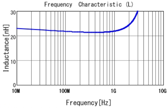
■ LQW15AN22NJ0Z L
