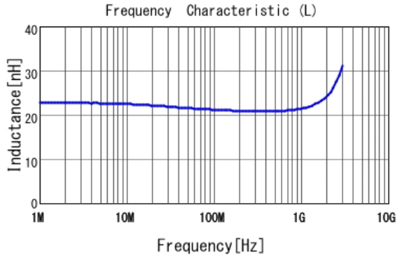
■ LQW15AN21NG80 L
