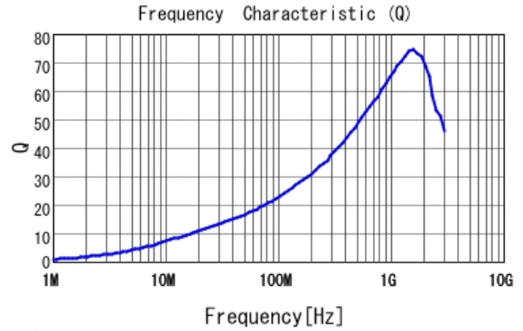
■ LQW15AN21NG80 Q
