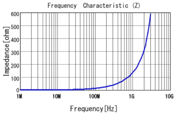
■ LQW15AN21NG80 |Z|
