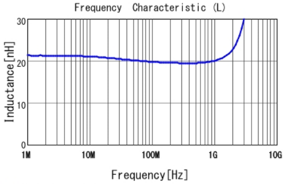
■ LQW15AN20NG80 L
