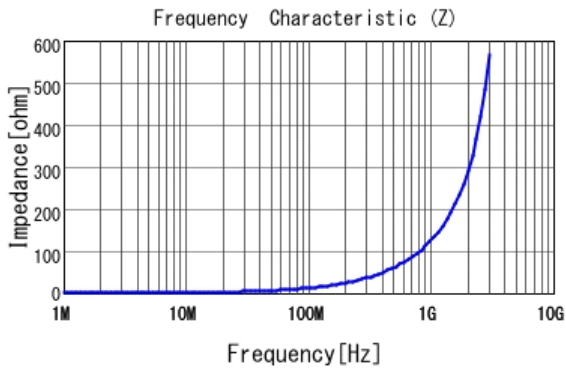
■ LQW15AN20NG80 |Z|
