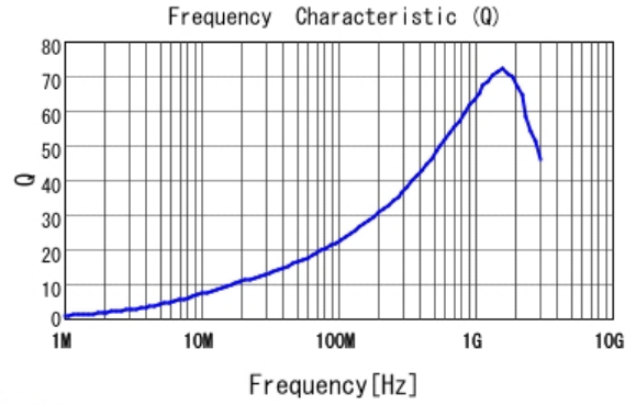
■ LQW15AN20NG80 Q
