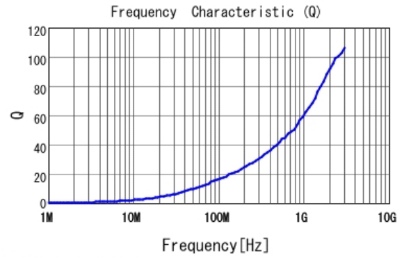
■ LQW15AN1N7C80 Q
