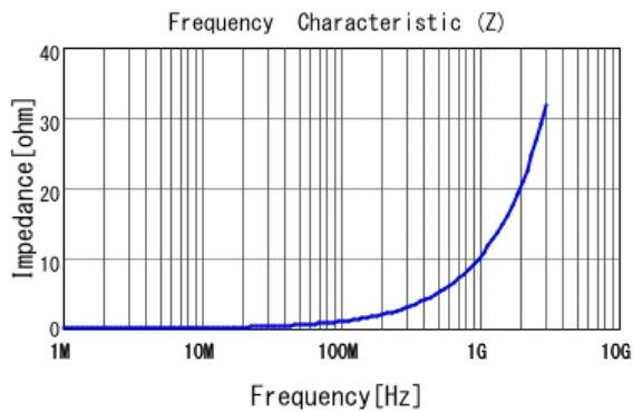
■ LQW15AN1N7C80 |Z|
