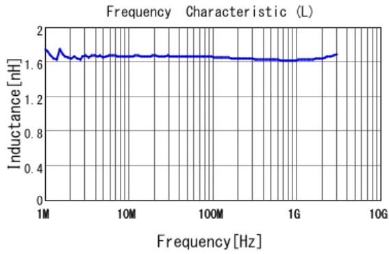
■ LQW15AN1N7C80 L
