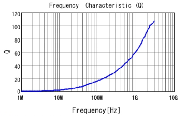
■ LQW15AN1N6C80 Q
