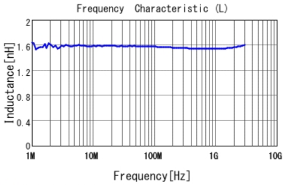
■ LQW15AN1N6C80 L
