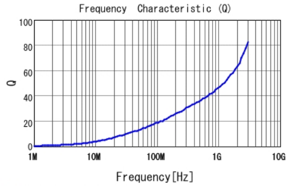
■ LQW15AN1N5D8Z Q
