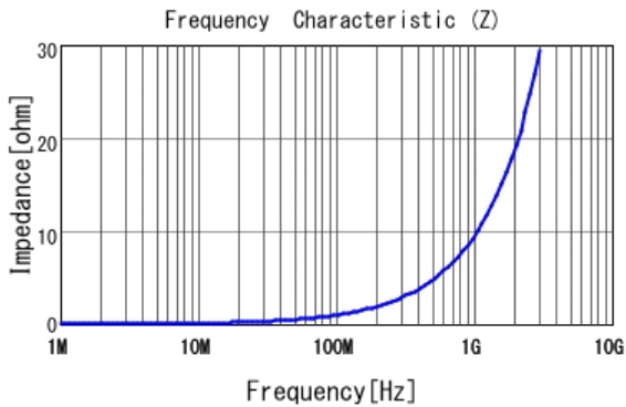
■ LQW15AN1N5D8Z |Z|
