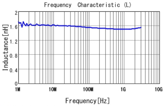
■ LQW15AN1N5D8Z L
