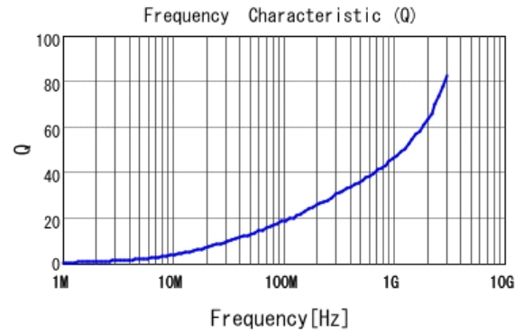
■ LQW15AN1N5D80 Q
