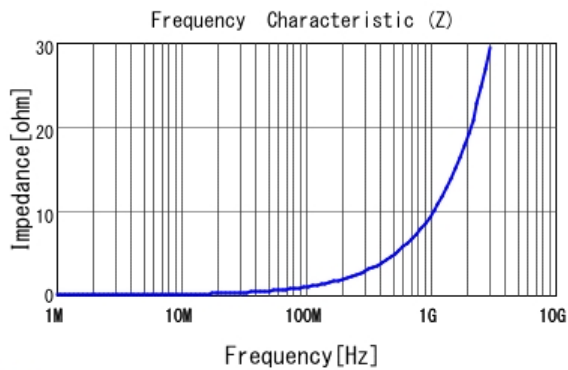
■ LQW15AN1N5D80 |Z|
