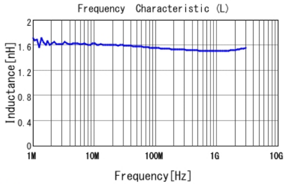
■ LQW15AN1N5D80 L
