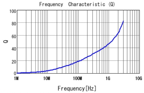
■ LQW15AN1N5C80 Q
