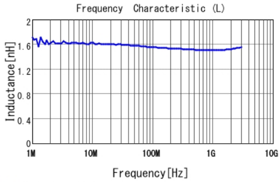
■ LQW15AN1N5C80 L
