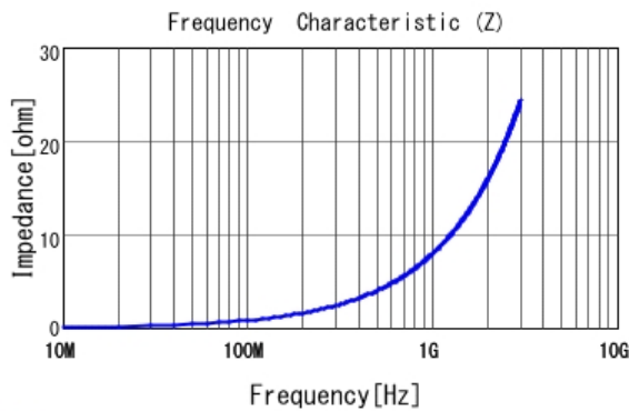
■ LQW15AN1N3D10 |Z|
