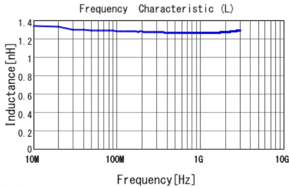
■ LQW15AN1N3D10 L
