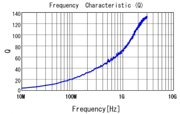
■ LQW15AN1N3D10 Q
