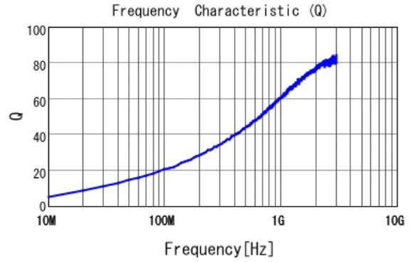
■ LQW15AN19NJ00 Q
