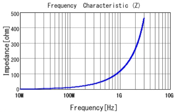
■ LQW15AN19NJ00 |Z|
