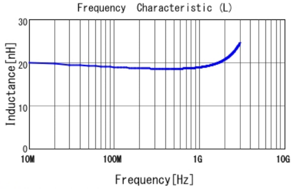
■ LQW15AN19NJ00 L
