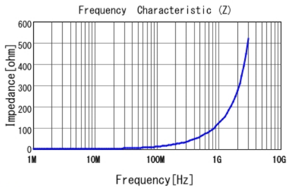
■ LQW15AN19NG80 |Z|
