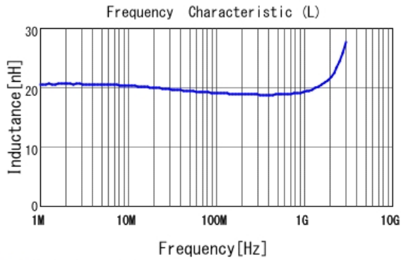
■ LQW15AN19NG80 L
