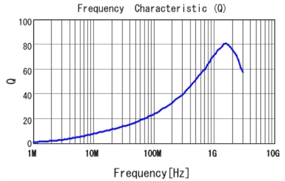
■ LQW15AN19NG80 Q
