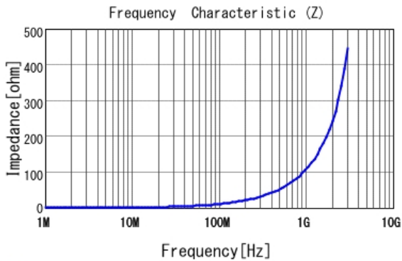
■ LQW15AN17NG80 |Z|
