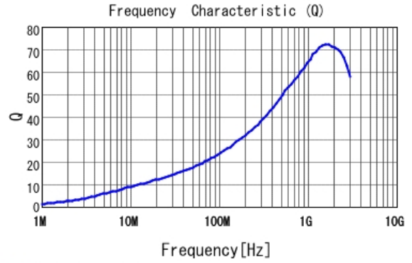
■ LQW15AN17NG80 Q
