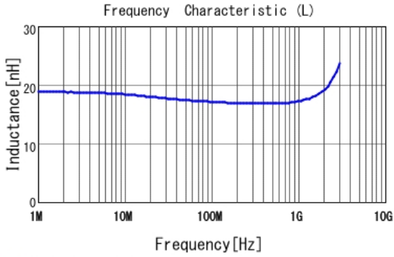
■ LQW15AN17NG80 L
