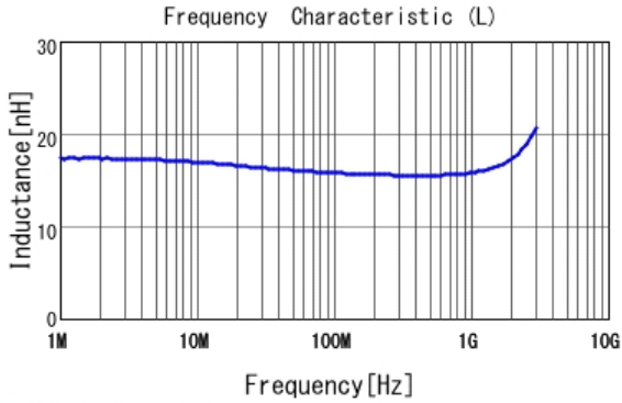
■ LQW15AN16NG8Z L
