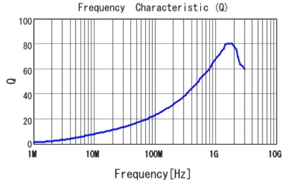
■ LQW15AN16NG8Z Q
