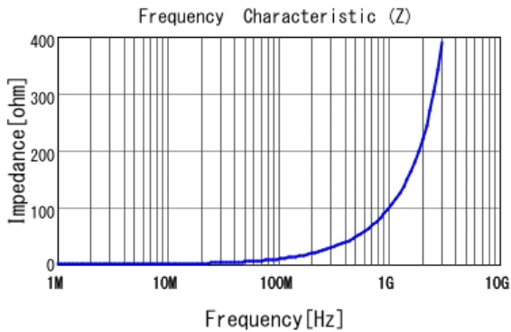
■ LQW15AN16NG8Z |Z|
