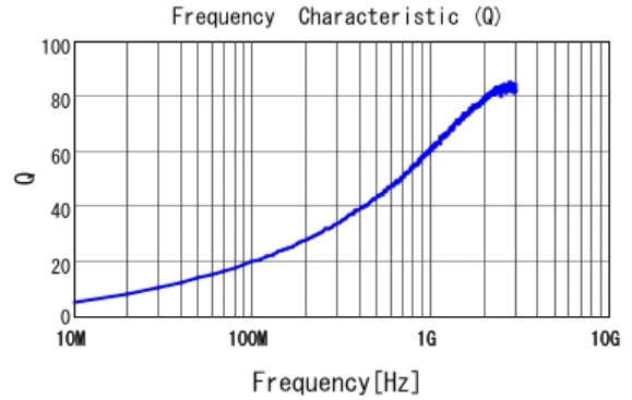
■ LQW15AN16NG0Z Q
