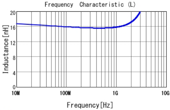
■ LQW15AN16NG0Z L
