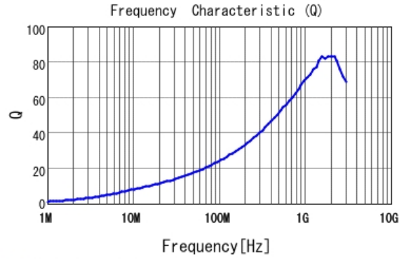
■ LQW15AN15NG8Z Q
