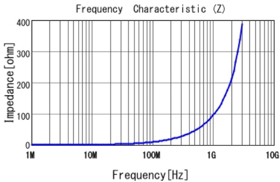
■ LQW15AN15NG8Z |Z|
