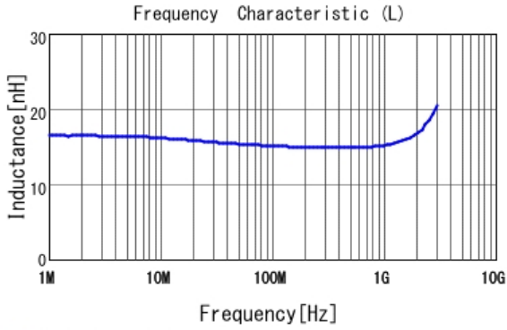
■ LQW15AN15NG8Z L
