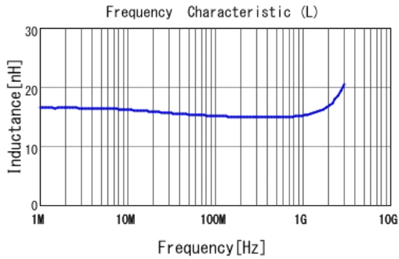
■ LQW15AN15NG80 L
