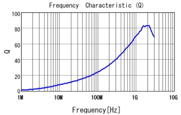
■ LQW15AN15NG80 Q
