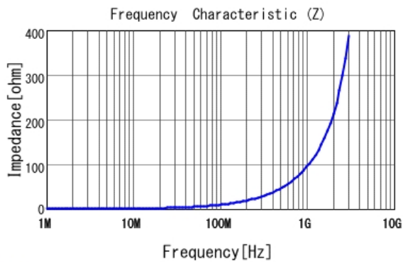
■ LQW15AN15NG80 |Z|
