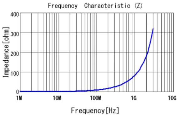
■ LQW15AN13NG8Z |Z|
