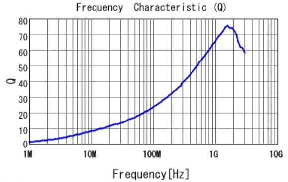
■ LQW15AN13NG8Z Q
