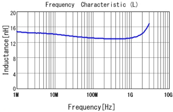
■ LQW15AN13NG8Z L
