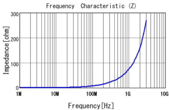
■ LQW15AN12NG80 |Z|
