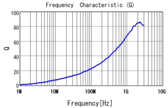
■ LQW15AN12NG80 Q
