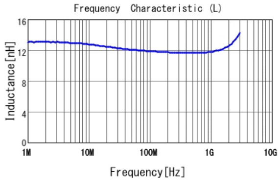
■ LQW15AN12NG80 L
