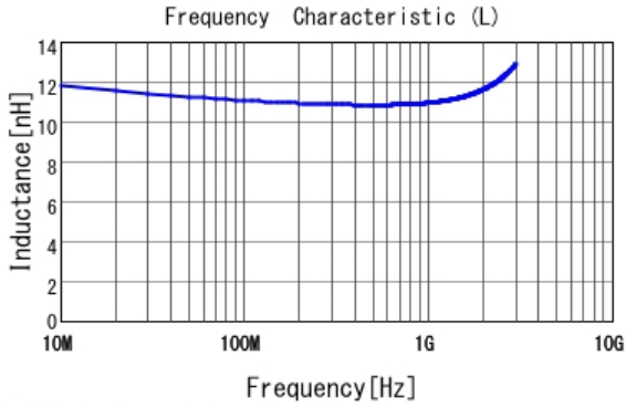
■ LQW15AN11NH00 L
