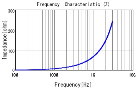
■ LQW15AN11NH00 |Z|
