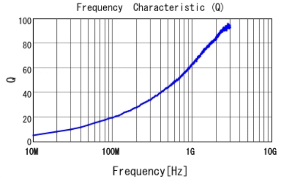
■ LQW15AN11NH00 Q
