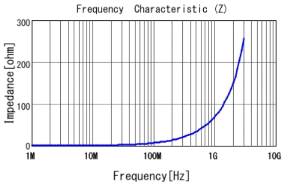
■ LQW15AN11NG80 |Z|
