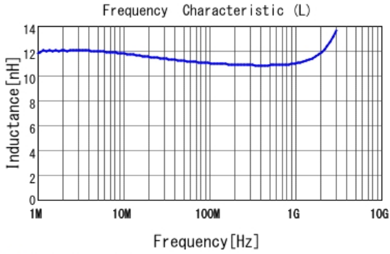
■ LQW15AN11NG80 L
