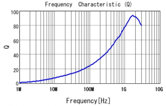
■ LQW15AN11NG80 Q
