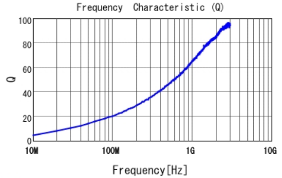
■ LQW15AN10NJ0Z Q
