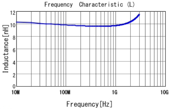
■ LQW15AN10NJ0Z L
