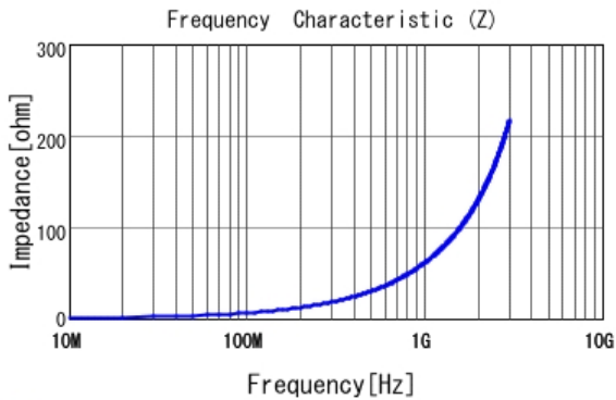
■ LQW15AN10NJ0Z |Z|
