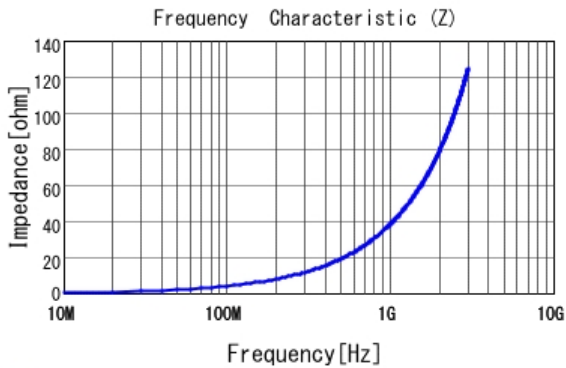
■ LQW04AN6N2D00 |Z|
