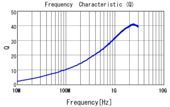
■ LQP03TQ8N2H02 Q
