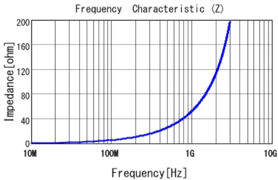
■ LQP03TQ8N2H02 |Z|
