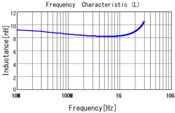
■ LQP03TQ8N2H02 L
