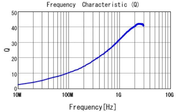
■ LQP03TQ7N5H02 Q
