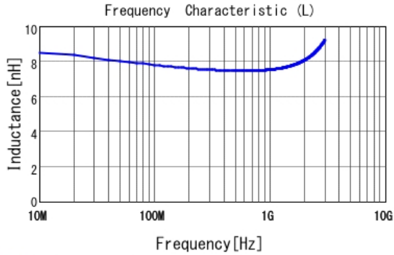
■ LQP03TQ7N5H02 L
