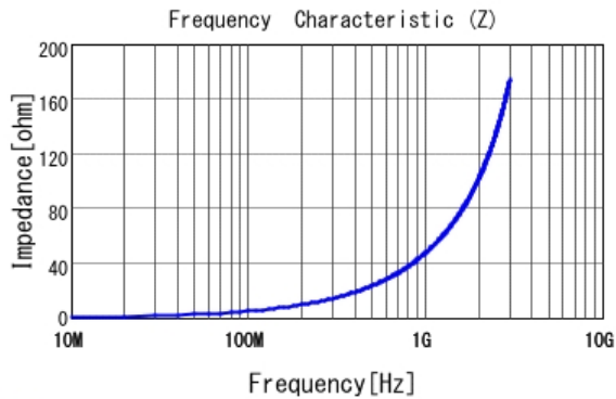
■ LQP03TQ7N5H02 |Z|
