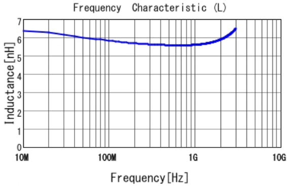
■ LQP03TQ5N6H02 L
