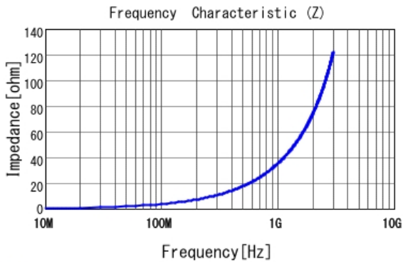
■ LQP03TQ5N6H02 |Z|
