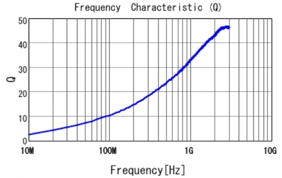
■ LQP03TQ5N6H02 Q
