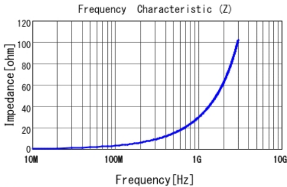
■ LQP03TQ4N7H02 |Z|
