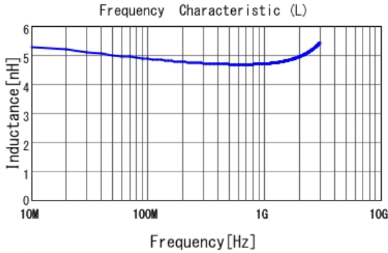
■ LQP03TQ4N7H02 L
