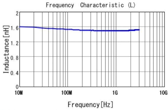
■ LQP03TQ1N5B02 L
