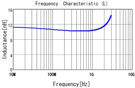
■ LQP03TQ10NJ02 L
