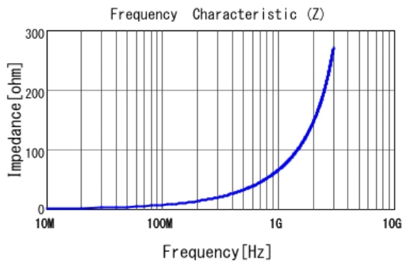
■ LQP03TQ10NH02 |Z|
