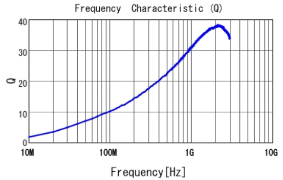
■ LQP03TQ10NH02 Q
