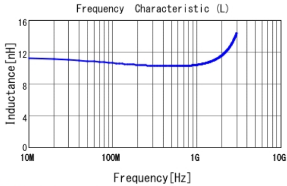
■ LQP03TQ10NH02 L
