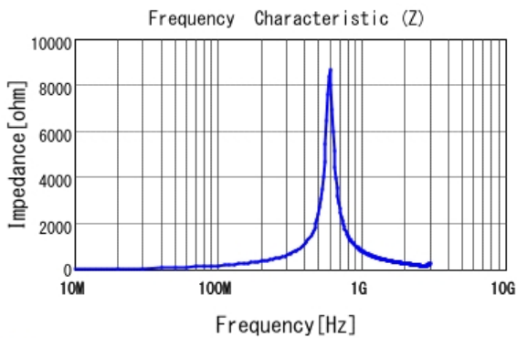
■ LQP03TNR27H02 |Z|
