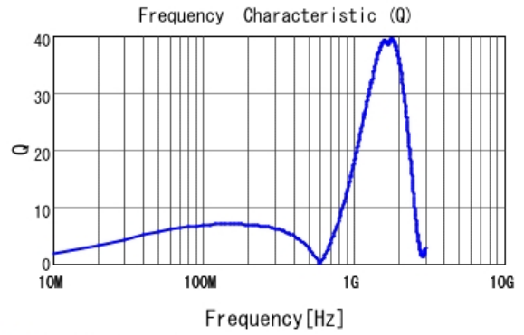
■ LQP03TNR27H02 Q
