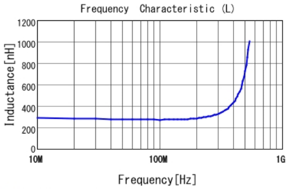
■ LQP03TNR27H02 L
