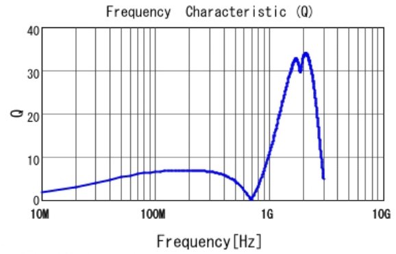
■ LQP03TNR22H02 Q
