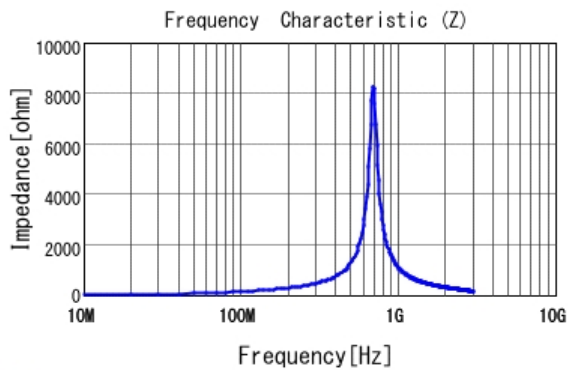
■ LQP03TNR22H02 |Z|
