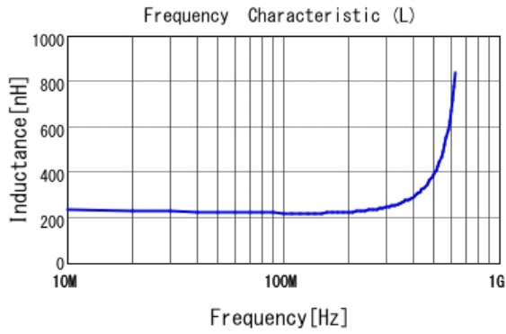
■ LQP03TNR22H02 L
