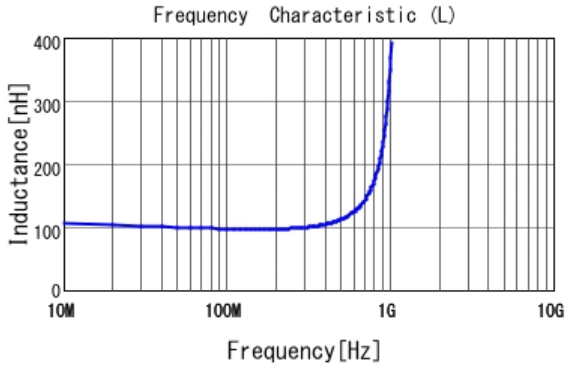
■ LQP03TNR10H02 L
