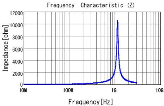
■ LQP03TNR10H02 |Z|
