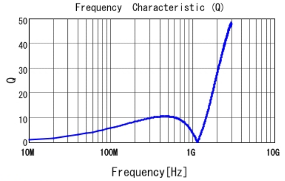
■ LQP03TNR10H02 Q
