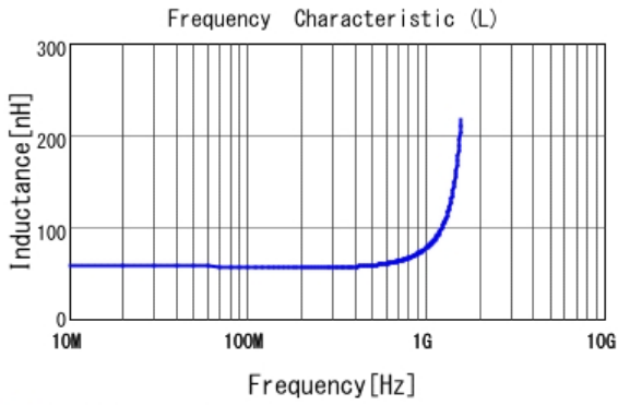
■ LQP03TN56NH02 L
