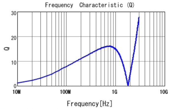
■ LQP03TN56NH02 Q
