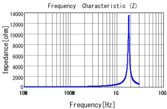
■ LQP03TN56NH02 |Z|
