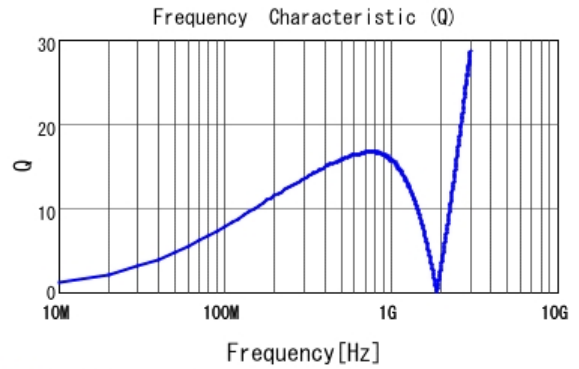
■ LQP03TN47NH02 Q
