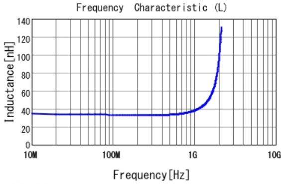
■ LQP03TN33NH02 L
