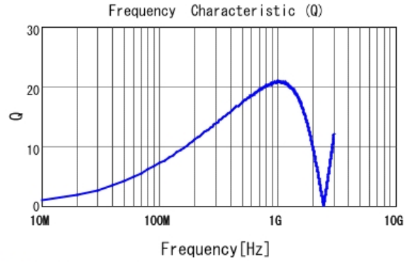
■ LQP03TN33NH02 Q
