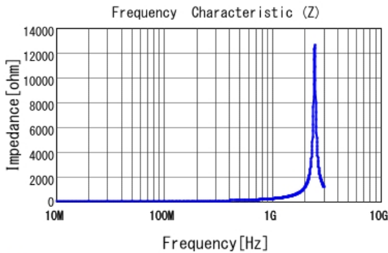
■ LQP03TN33NH02 |Z|
