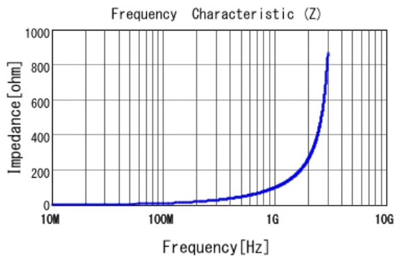
■ LQP03TN15NHZ2 |Z|
