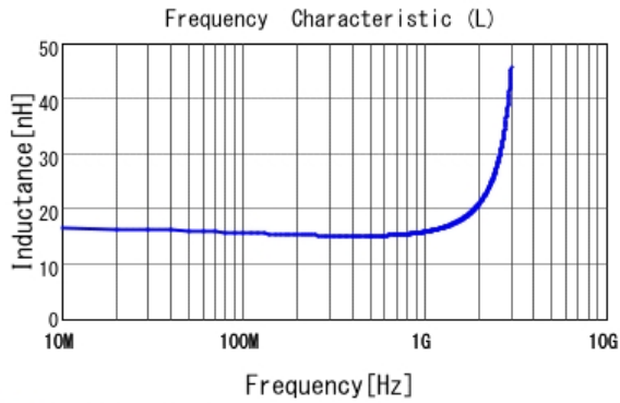
■ LQP03TN15NHZ2 L
