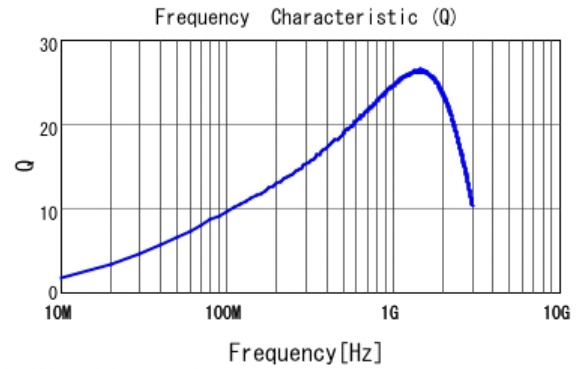
■ LQP03TN15NHZ2 Q
