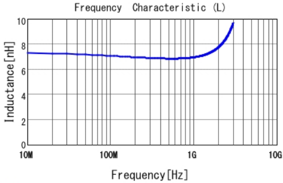
■ LQP03TG6N8H02 L
