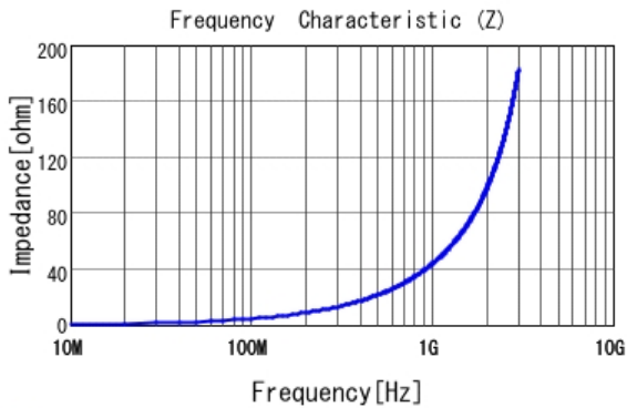
■ LQP03TG6N8H02 |Z|
