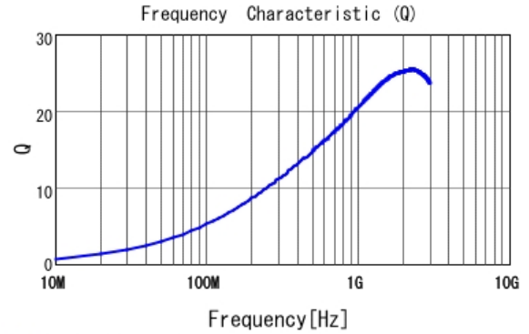
■ LQP03TG6N8H02 Q
