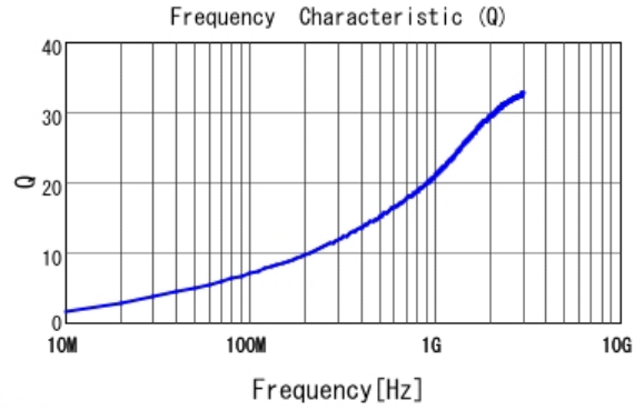
■ LQP03TG2N2B02 Q
