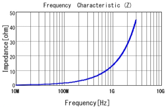
■ LQP03TG2N2B02 |Z|
