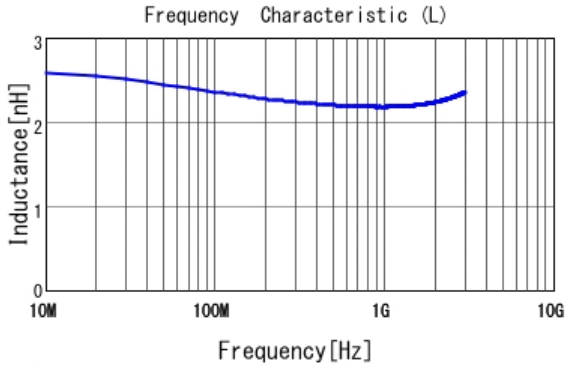
■ LQP03TG2N2B02 L
