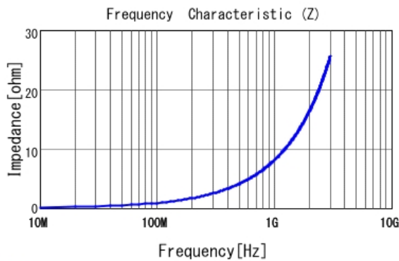
■ LQP03TG1N3B02 |Z|
