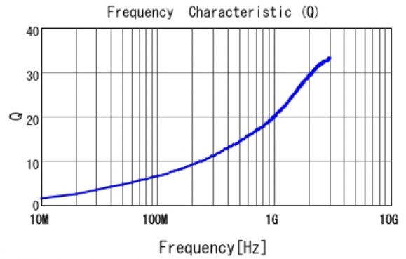
■ LQP03TG1N3B02 Q
