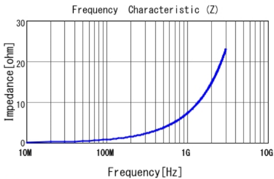
■ LQP03TG1N2B02 |Z|
