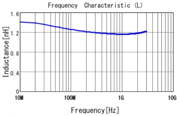
■ LQP03TG1N2B02 L
