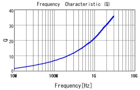
■ LQP03TG1N2B02 Q
