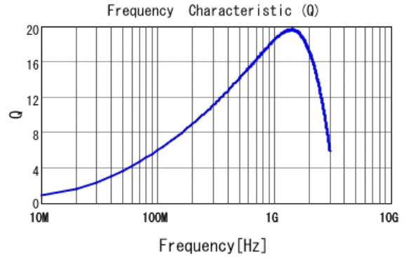
■ LQP03TG15NH02 Q
