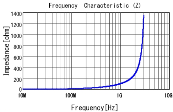
■ LQP03TG15NH02 |Z|
