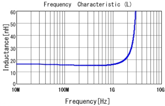
■ LQP03TG15NH02 L
